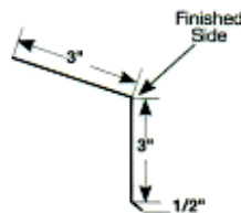
Eave 3x3x1/2 KO
