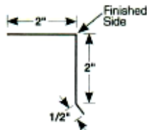
Drip Edge 2x2x1/2 KO
